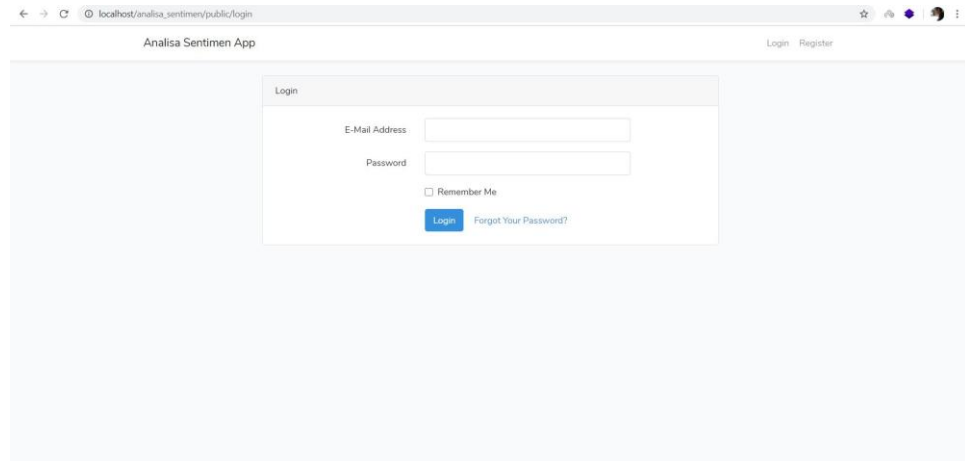
Gambar 5.2 Implementasi Login.
